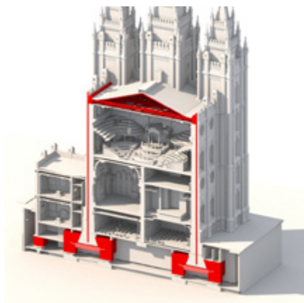
Ang gisugyot nga pagpalig-on sa Templo sa Salt Lake alang sa linog gikonsiderar nga maoy labing bag-o nga engineering alang sa proteksyon batok sa linog.
